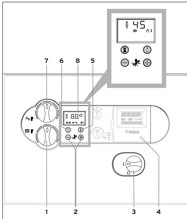
Рис. 4.2 Элементы управления
